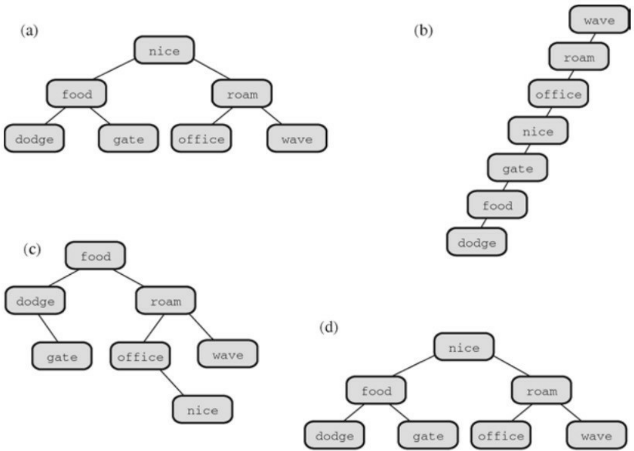
图A.1 单词的二分查找树
