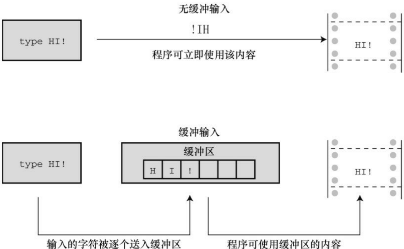
图8.1 缓冲输入和无缓冲输入
