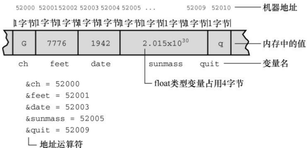
图9.6 按字节寻址系统（如PC）中变量的名称、地址和值
