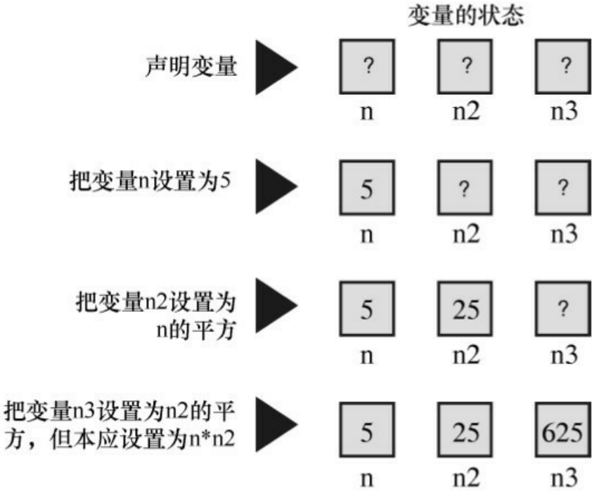
图2.6 跟踪程序的执行步骤
