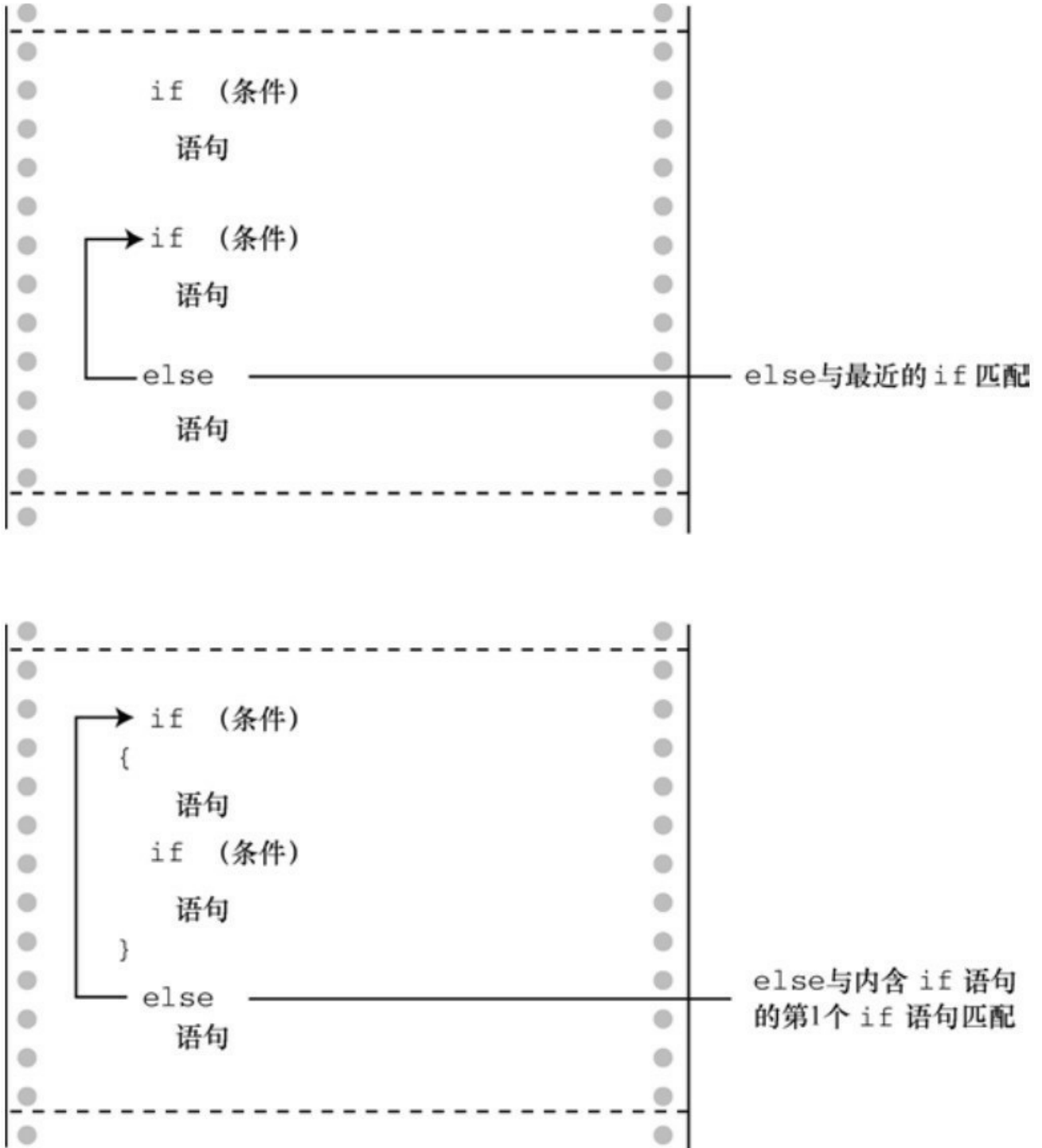
图7.2 if else匹配的规则
