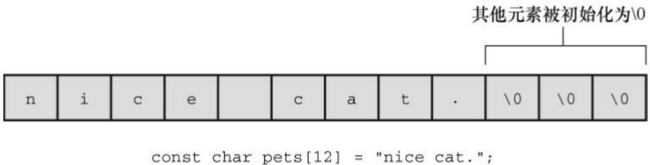
图11.1 初始化数组
