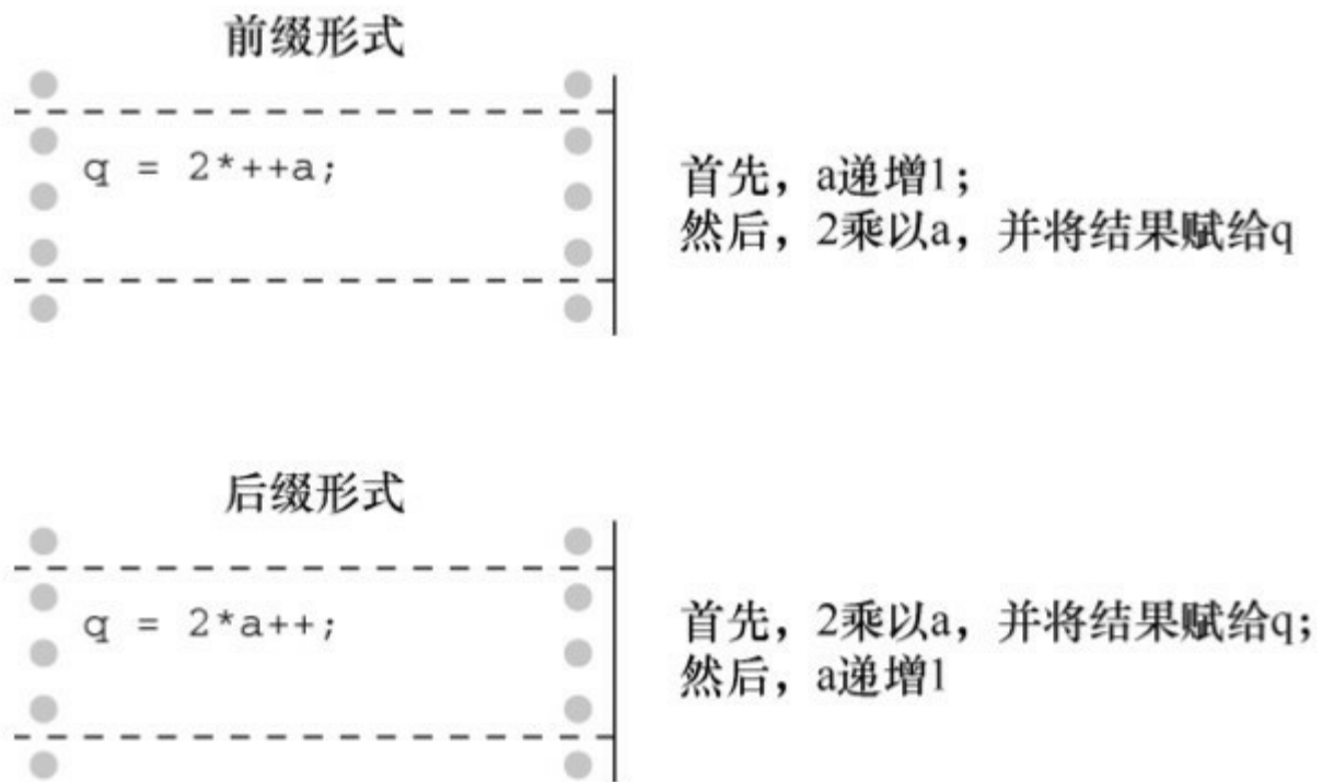
图5.5 前缀和后缀
