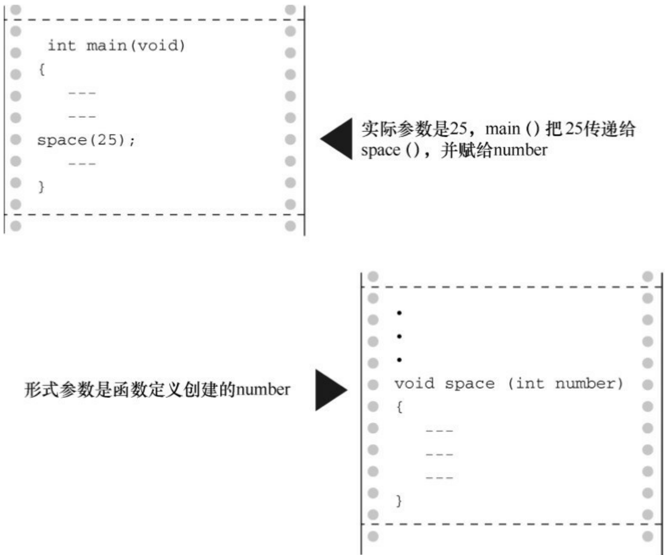
图9.3 形式参数和实际参数
