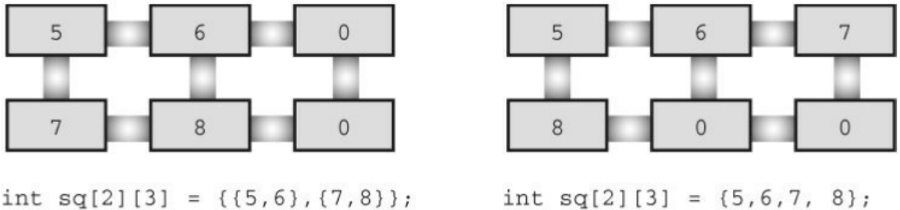
图10.2 初始化二维数组的两种方法
