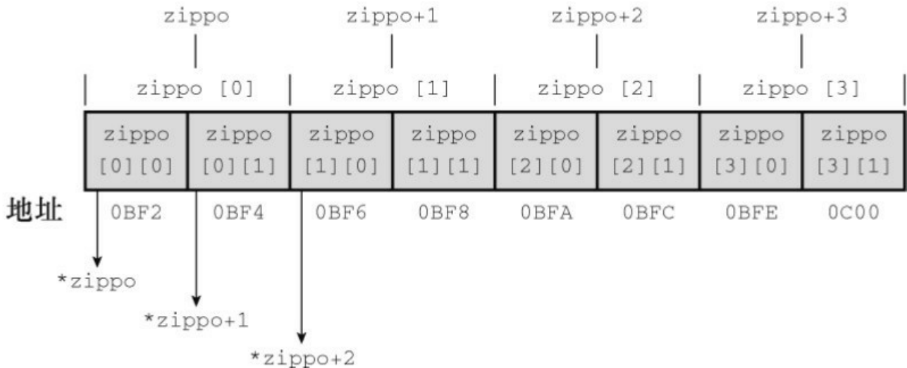
图10.5 数组的数组
