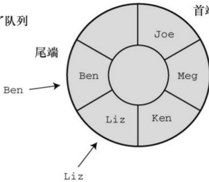
图17.8 环形队列
