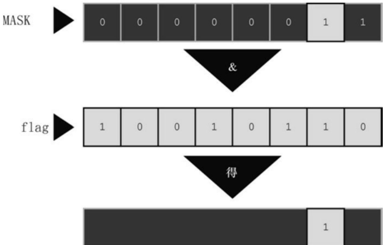
图15.2 掩码示例
