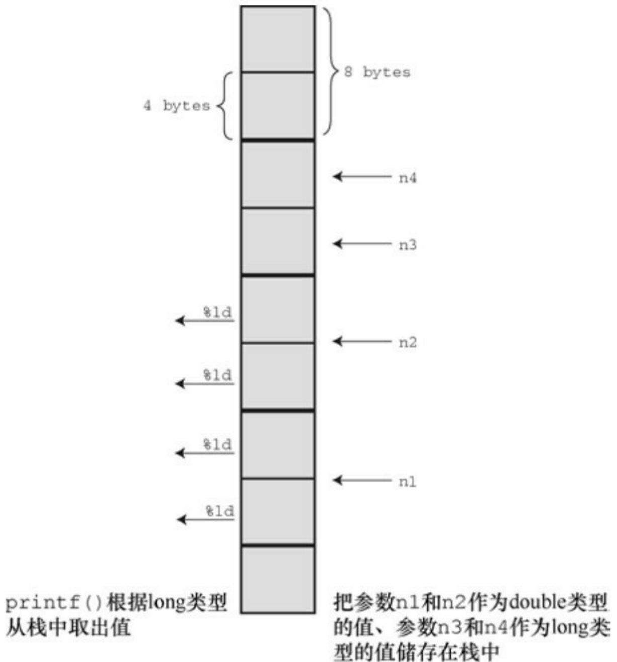
图4.9 传递参数
