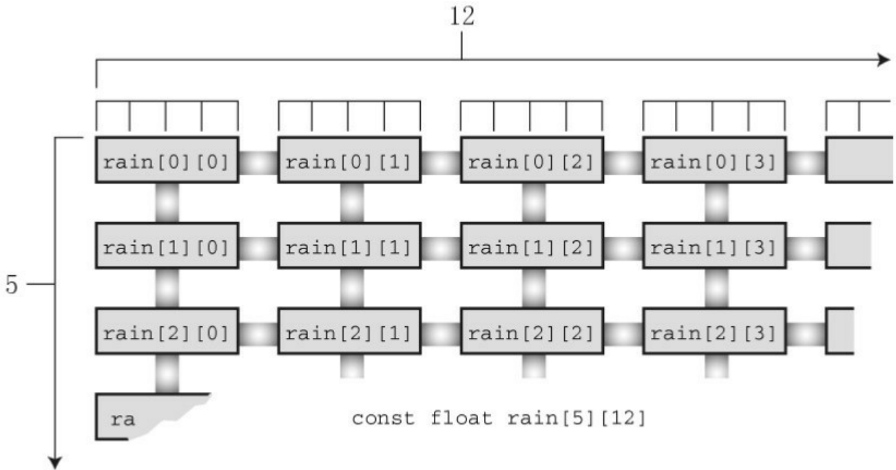
图10.1 二维数组
