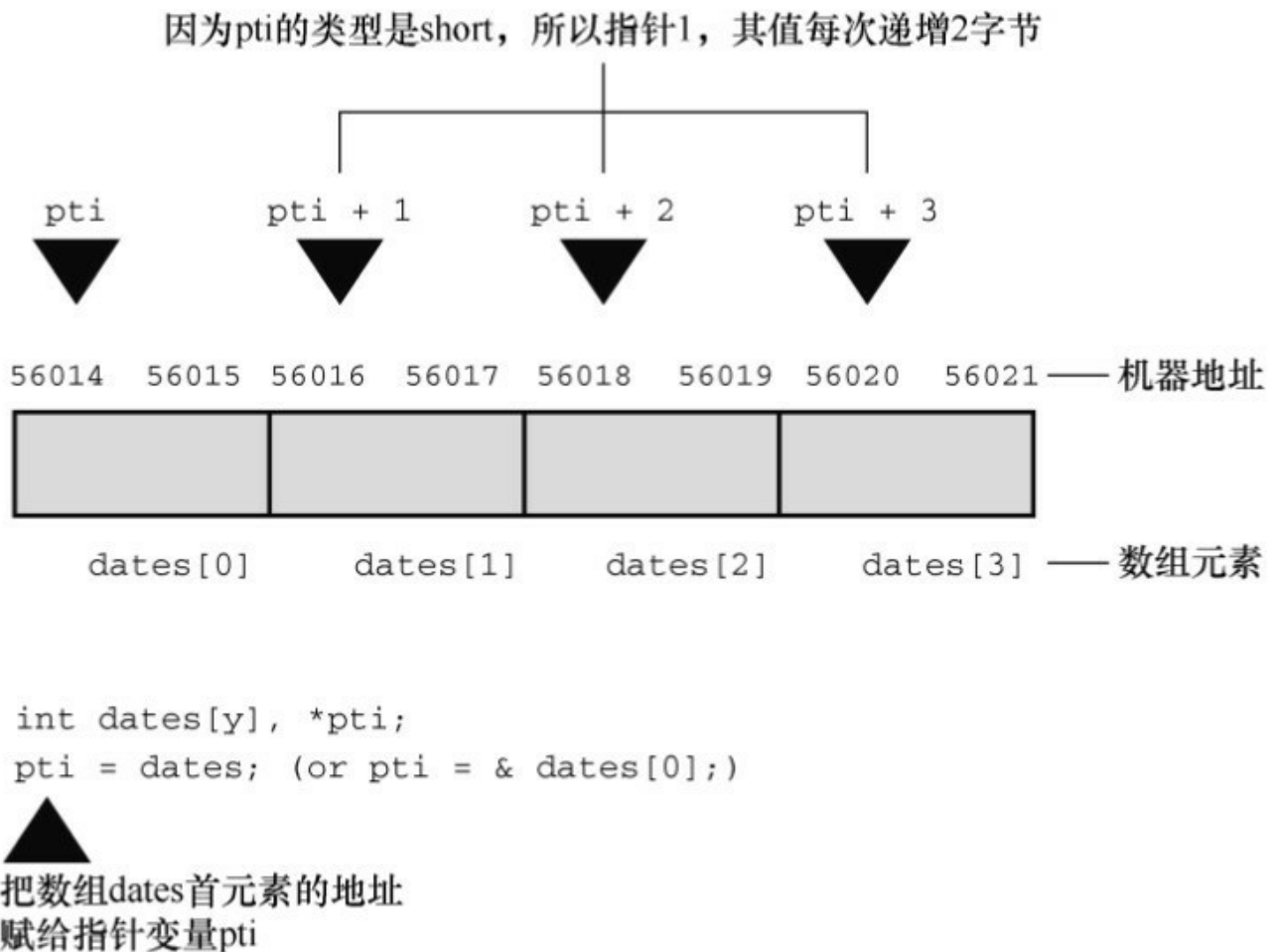
图10.3 数组和指针加法
