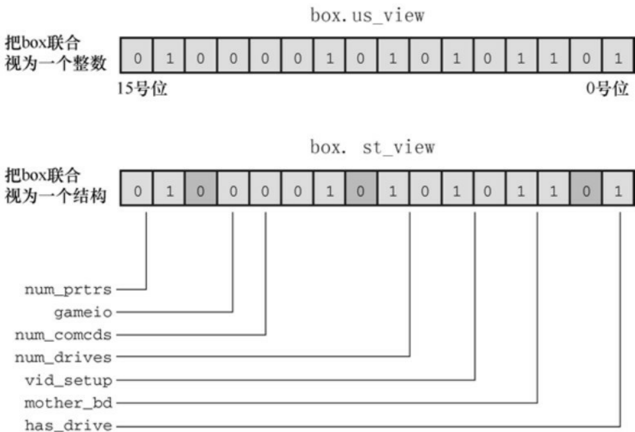
图15.3 作为整数和结构的联合
